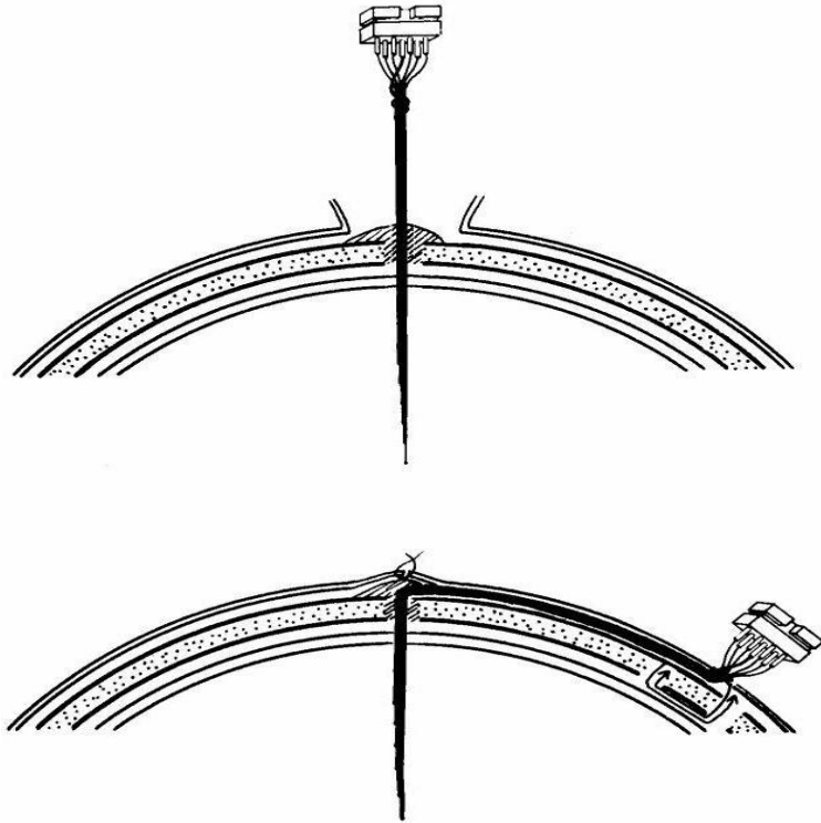
Illustration 1: Schéma du montage d'une électrode implantée dans le cerveau et ancrée au crâne. Les profondeurs du cerveau sont ainsi accessibles en branchant simplement un connecteur (52).
