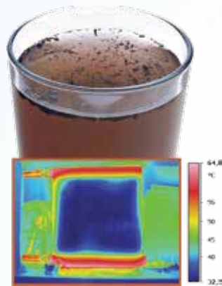
Radiateur emboué
