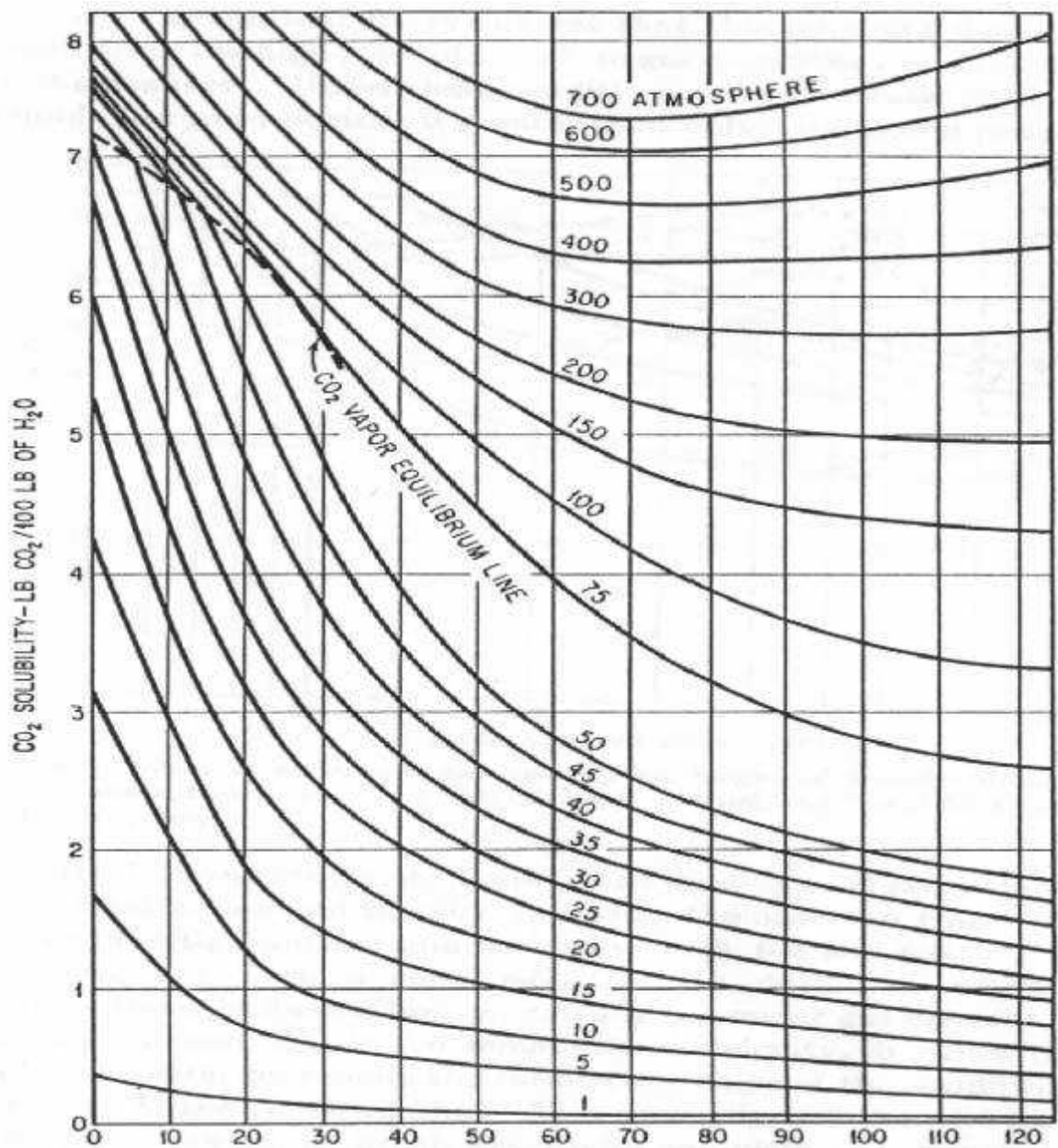
Figure 5 : Solubilité du CO 2 dans l'eau en fonction de la température en °C (Khol et Nielsen, 1997)
