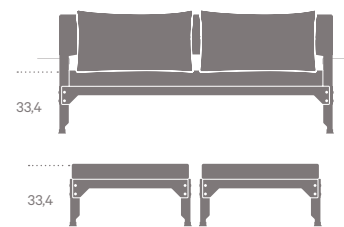
Canapé farniente Farniente sofa
