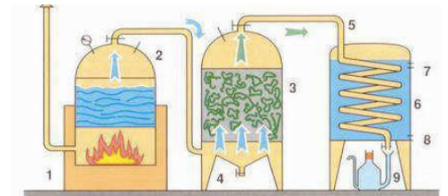
1. Foyer - 2. Chaudière - 3. Vase à fleurs - 4. Vidange de condensation - 5. Col de cygne 6. Réfrigérant avec serpentin 7. Sortie d'eau chaude - 8. Arrivée d'eau froide - 9. Essencier servant à la décantation de l'essence et de l'hydrolat
