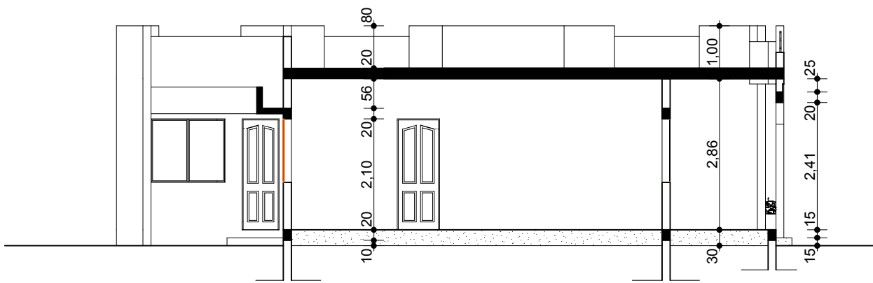
Coupe B-B Echelle : 1/100
