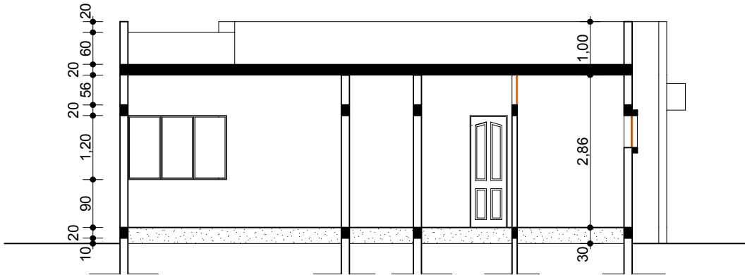
Coupe A-A Echelle : 1/100
