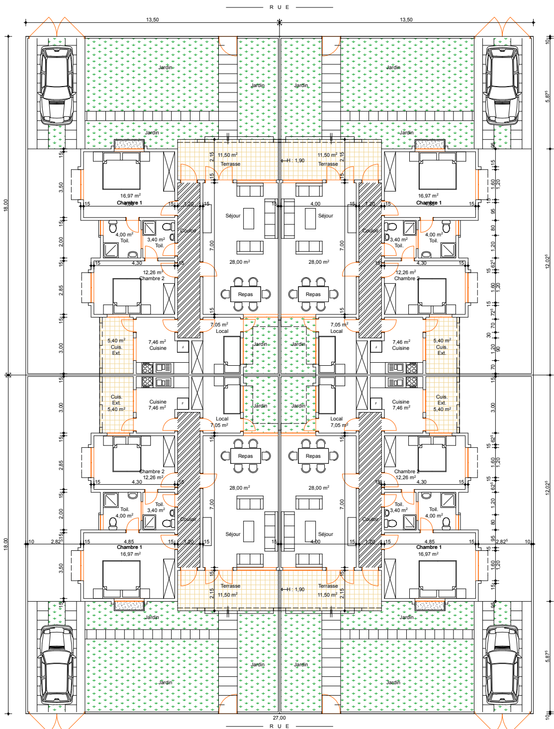
Vue en Plan Aménagé - Côté ( Quatre Appartements Type F3 plus regroupés )
