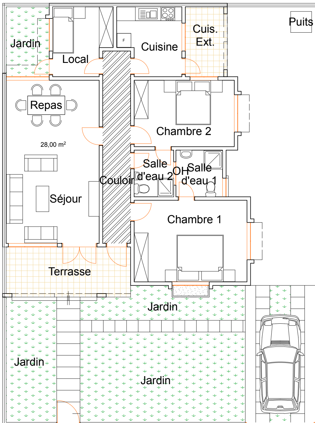
Plan Aménagé ( Type F3 plus ) R U F Échelle: 1/50
